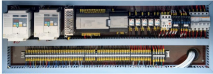
Boitier Electrique
